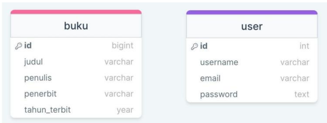
Gambar 1. Desain Konseptual Database Soal 1 Modul 7
